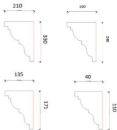
ACE-M25 G2 330x210 - No.16
